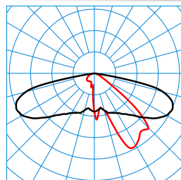
Publisca P2-AB2L/2000-740 3G1S TX047709 ■ C0 - C180 ■ C90 - C270 DIN 5040: A30 UTE: 1,00 l DLOR: 100 % ULOR: 0 % CEN Flux Code: 34 71 96 100 100
