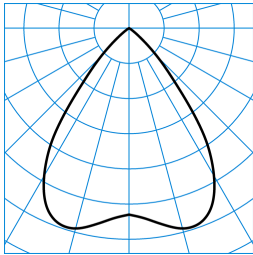
InperiaL G2 C07 BR19 1800-830 ET 03 ■ C0 - C180 TX0528190
