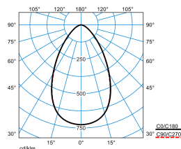
E-Line PRO 78IP50 MironaF TB 200-840 ET L150 01 01 (LEO2)
