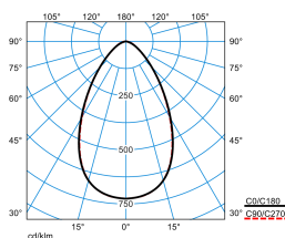
E-Line PRO 78IP50 MironaF TB 200-840 ET L150 01 Blank (LE01)
