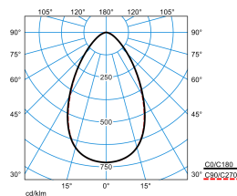
E-Line PRO 78IP50 MironaF TB 200-840 ET L150 01 Blank (LEO2)
