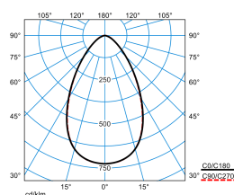
E-Line PRO 78IP50 MironaF TB 200-840 ET L150 01 Blank IP50 (LEO1)
