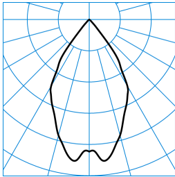
InperiaLP C05 BR22 2700-830 ET 01 ■ C0 - C180 TX771492
