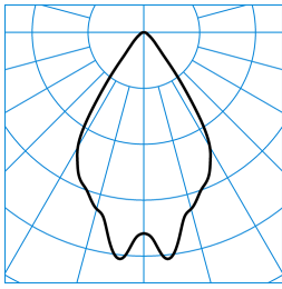
InperiaLP C05 BR22 2700-830 01 + RG-PC TX041561 ■ C0 - C180
