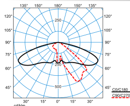
Publisca P2-AB2L/4200-730 6G1S TX047724 DIN 5040: A30 UTE: 1,00 G DLOR: 100 % ULOR: 0 % CEN Flux Code: 35 74 97 100 100
