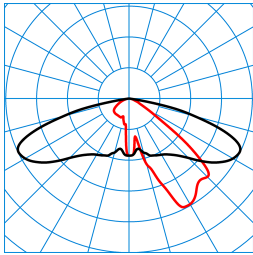
Publisca P2-AB2L/4200-730 6G1S ETDD (CLO end value) TX300238 ■ C0 - C180 ■ C90 - C270 DIN 5040: A30 UTE: 1,00 G DLOR: 100 % ULOR: 0 % CEN Flux Code: 35 74 97 100 100
