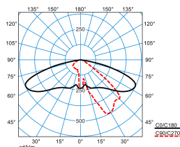
Publisca P2-AB2L/4200-730 6G1S ETDD (CLO end value) TX300238 DIN 5040: A30 UTE: 1,00 G DLOR: 100 % ULOR: 0 % CEN Flux Code: 35 74 97 100 100
