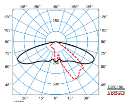
Publisca P2-AB2L/4200-730 6G1S ETDD (CLO initial value) TX301116 DIN 5040: A30 UTE: 1,00 G DLOR: 100 % ULOR: 0 % CEN Flux Code: 35 74 97 100 100
