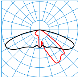
Publisca P2-AB2L/4200-730 6G1S TX047724 ■ C0 - C180 ■ C90 - C270 DIN 5040: A30 UTE: 1,00 G DLOR: 100 % ULOR: 0 % CEN Flux Code: 35 74 97 100 100
