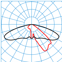
Publisca P2-AB2L/4200-730 6G1S ETDD (CLO initial value) TX301116 ■ C0 - C180 ■ C90 - C270 DIN 5040: A30 UTE: 1,00 G DLOR: 100 % ULOR: 0 % CEN Flux Code: 35 74 97 100 100
