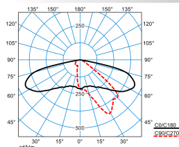
Publisca P3-AB2L-LRA/3200-730 4G1 ET (CLO initial value)
