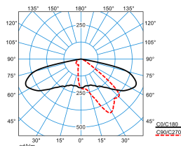
Publisca P3-AB2L-LRA/2200-730 4G1
