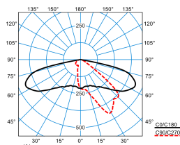
Publisca P3-AB2L-LRA/2200-730 4G1 ET (CLO end value)
