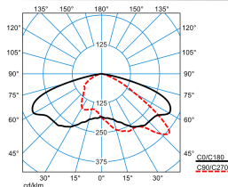
LnPlus 40-AB7L-SLR2/5100-740 6G1 ET (CLO initial value)
