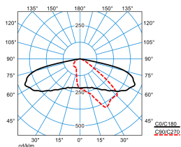
LIQ 50N-AB2L-LR/6800-727 6G1 ET (CLO end value)
