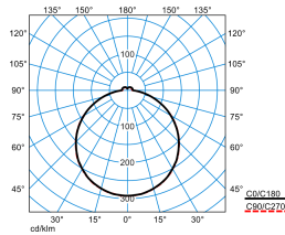
Olisq QWD3 DW 45-840 ET IP54 IK
