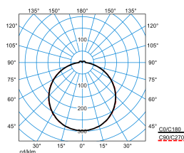
Olisq QWD3 DW 45-840 ET IP54 IK + Olisq QWD3 ZDR 1/2 03
