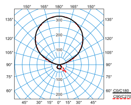
Luceos S-T PAW-IL 300-840 ETDD 01 (LEO1)
