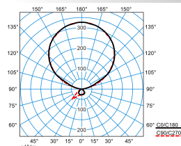
Luceos S-T PAW-IL 300-840 ETDD 01 (LEO2)
