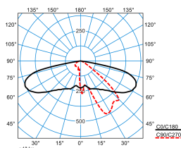
Publisca P1-AB2L-LR/2400-730 3G1S ET (CLO end value) TX301759 DIN 5040: A30 UTE: 1,00 l DLOR: 100 % ULOR: 0 % CEN Flux Code: 34 71 96 100 100
