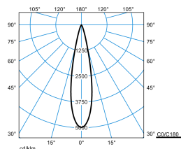
E-Line PRO 78 Lentyp L-SP 20-840 M35 ET 05 05
