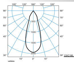
E-Line PRO 78 BV G2 RF-FL 20-840 M35 ET 05 Blank
