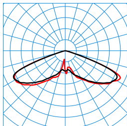
Publisca P1-RB6L-LR/2400-740 3G1S ET (CLO end value) TX300260 ■ C0 - C180 ■ C90 - C270 DIN 5040: A20 UTE: 1,00 J DLOR: 100 % ULOR: 0 % CEN Flux Code: 20 57 98 100 100
