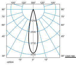
E-Line PRO 78 LentyP L-SP 40-830 M33 ET 01 TX715067
