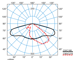
LnPlus 40-AB7L-LR/13500-727 12G1 ET (CLO end value) TX377032
