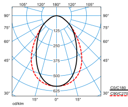
ArimoFit G2 M59 DW19 53-840 ET TX376381
