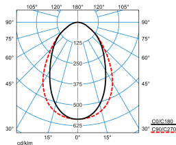
ArimoFit G2 M59 DW19 53-840 ET + ArimoFit G2 Sky M59-TS ZER TX426814
