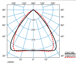
ELINE LN120 840 L225 1 20
