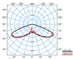
Publisca P2-RB6L-LR/2600-730 3G1S ET (CLO end value)
