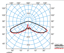
Publisca P2-RB6L-LR/2600-730 3G1S ET (CLO initial value)
