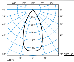
E-Line PRO 78 BV G2 RF-WFL 20-827 M32 ET 01 01
