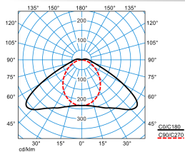
Nextrema G3 XB 4000-840 ET +LV TX770566
