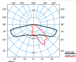
9301K AB2L-LR-SLR3/2900-740 4G3 ET (CLO initial value)
