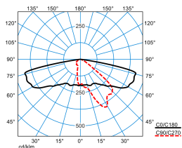
9301K AB2L-LR-SLR3/2900-740 4G3 ET (CLO end value)
