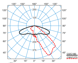
Publisca P2-AB2L-LR/3200-740 4G1S ET (CLO end value)
