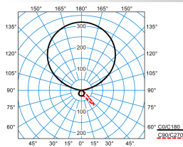
Luceos S G3 PAW-IL 170-8TW ETDS FU 03 (DWW)
