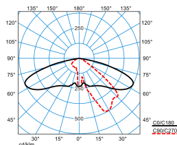
Publisca P2-AB2L/3800-740 6G1S ETDD (CLO end value)
