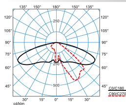
Publisca P2-AB2L/3800-740 6G1S
