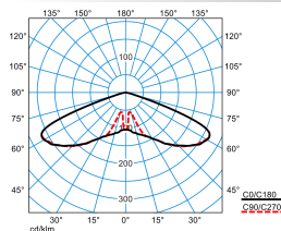
Publisca P2-RB6L-LR/1200-740 2G1S ET (CLO initial value)
