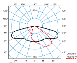
LIQ 70N-AB7L-SLR2/7500-722 8G1 ET (CLO end value)
