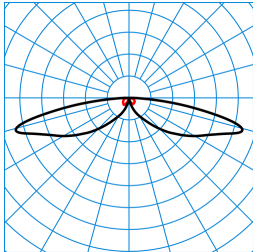
LTX KT-SB3L-LR/1500-730 2G1 ET TX780600
