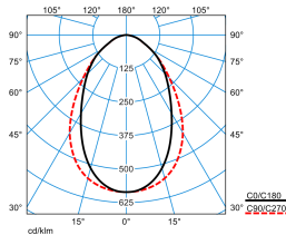
ArimoFit G2 M59 DW19 IP 53-840 ETDD TX376504
