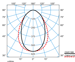
ArimoFit G2 M59 DW19 IP 53-840 ETDD + ArimoFit G2 Sky M59-TS ZER TX426817
