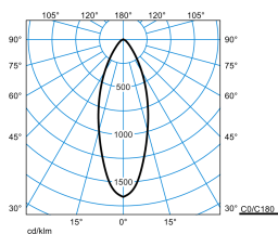
Amatris QC2 WRRFL 8-9MC ET 01 2KIT + PC IP54 (stage 1)
