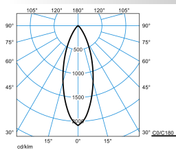
Amatris QC2 WRRFL 8-9MC ET 01 2KIT + HC-19 05 (stage 1)
