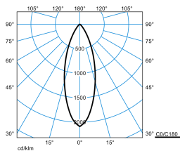
Amatris QC2 WRRFL 8-9MC ET 01 2KIT + HC-19 05 (stage 3)
