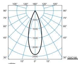
7651 LentyP L-FL 30-840 M35 ET 05 (225)
