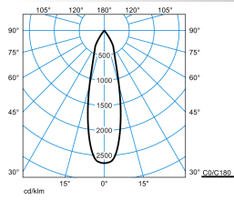
SisC 2Z RF-MF 2x50-830 M33 ETDD 05
