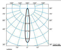
E-Line PRO 78 BV G2 RF-SP 20-BF M54 ET 03 03
