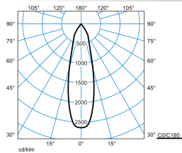
TaroMini 3PTD RF-MF 40-840 M35 ET 05
