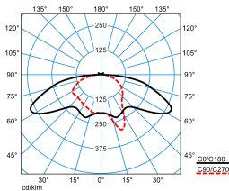
9851IA-LRA/2200-840 ET TX780726
