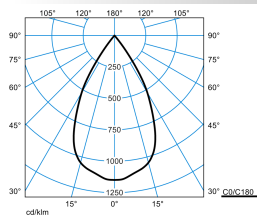
E-Line PRO 78 BV G2 RF-VFL 50-840 M35 ETDD 01 Blank
